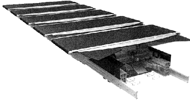
รูปที่ 1 ลักษณะของชุดสายพานรับสิ่งของแบบ Cross Belt
